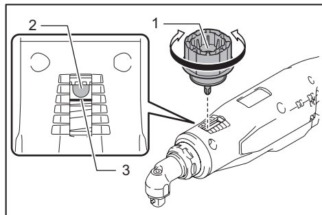
► 1. Manija de ajuste 2. Orificio para la manija de ajuste 3. Línea amarilla
